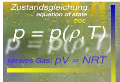
Abbildung 27.3: Mathematische Form von Zustandsgleichungen und ideales Gas.
