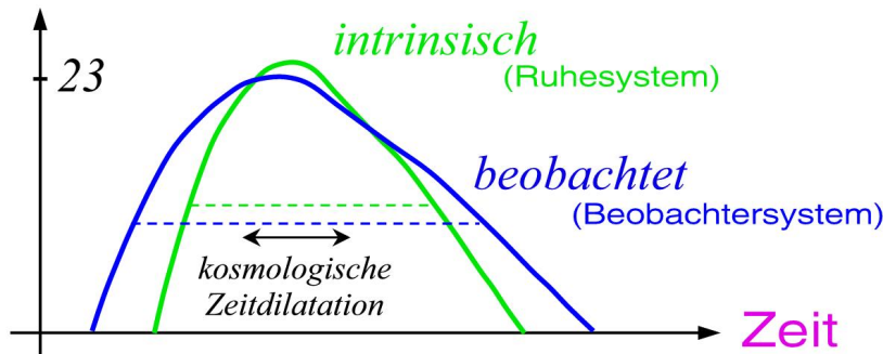
Abbildung 27.2: kosmologische Zeitdilatation in Supernova-Lichtkurven.
