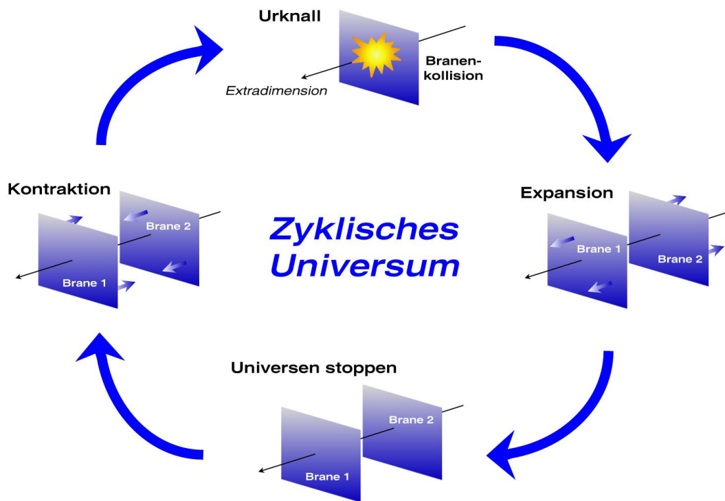
Abbildung 27.5: Stadien im Zyklischen Universum.
